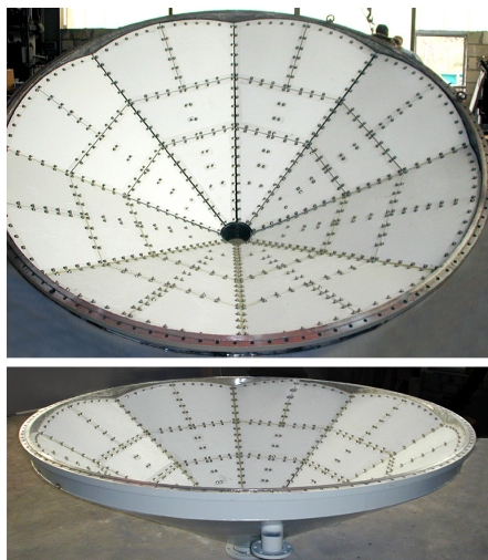
grand silo avec segments confectionnés
